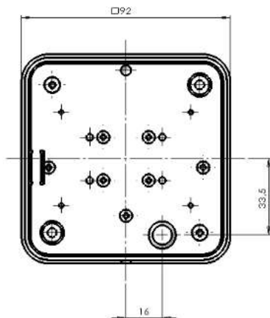
Måttavering styrenhet för kabelgenomföring från baksidan
