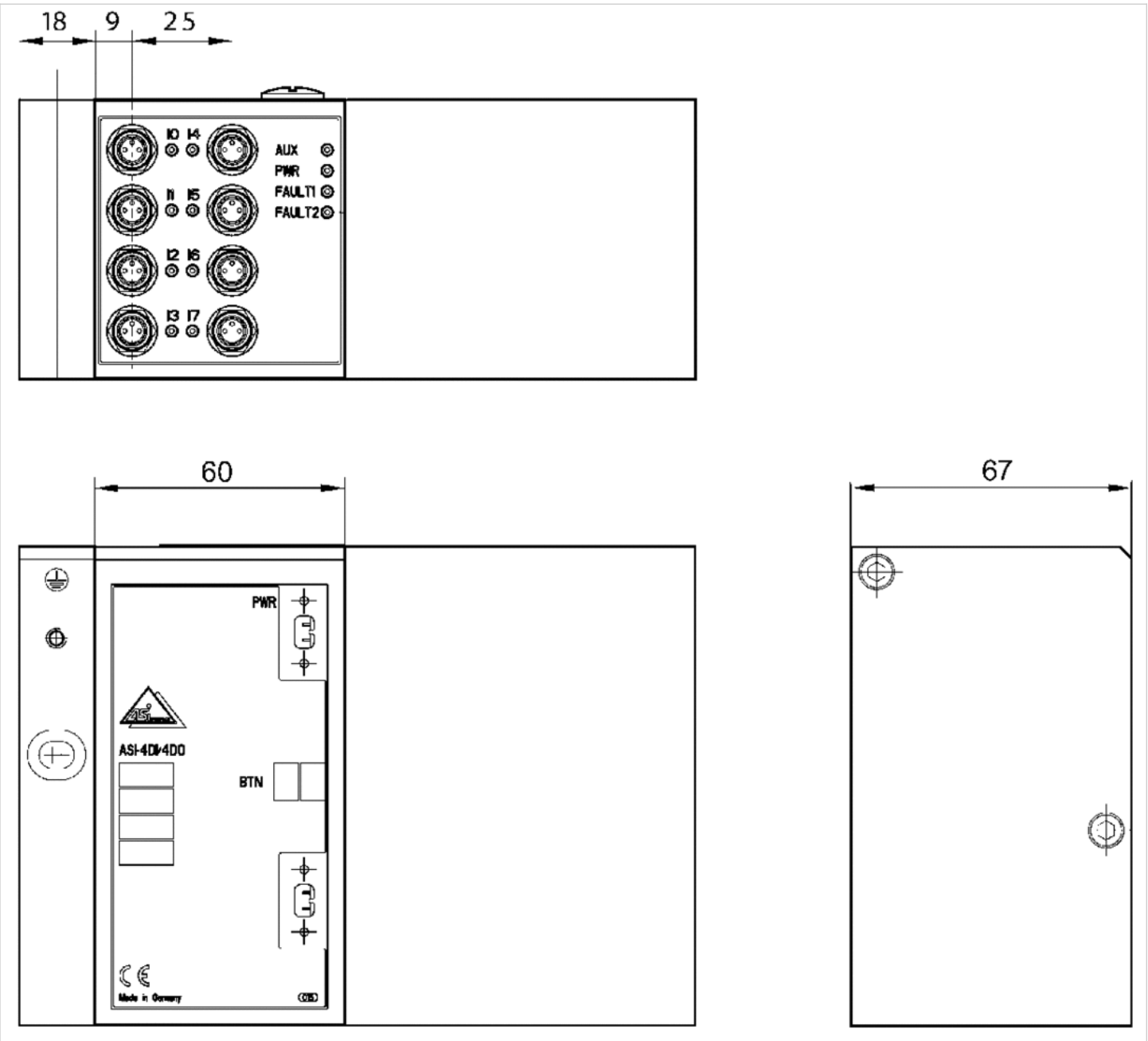
8DI/8DO-AUX
